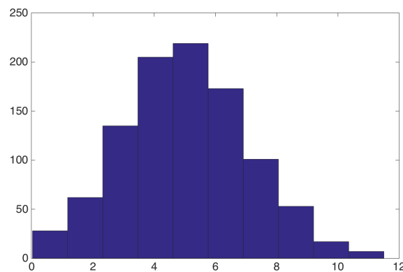
Figur 1: Histogram for observasjoner av sann gjennomstrømning ( x )
